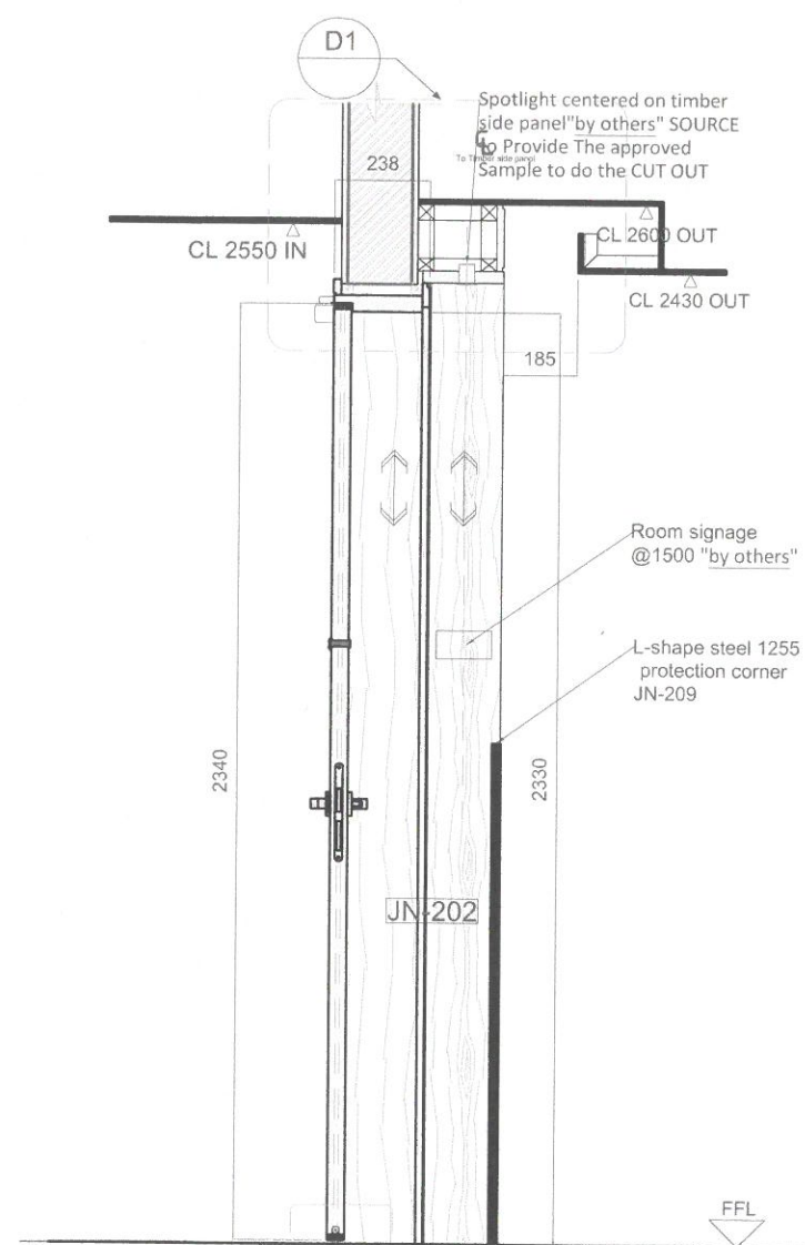
D2 Section
